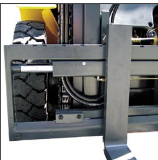
boční posuv vidlí
